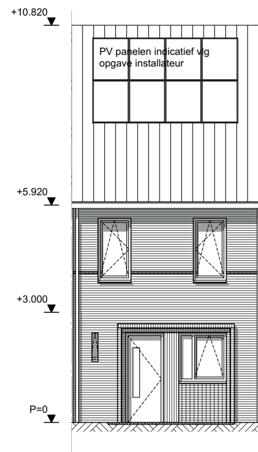
Voorgevel
