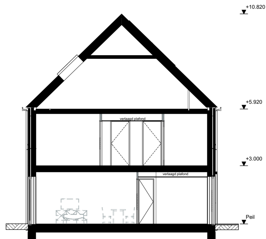
Doorsnede
