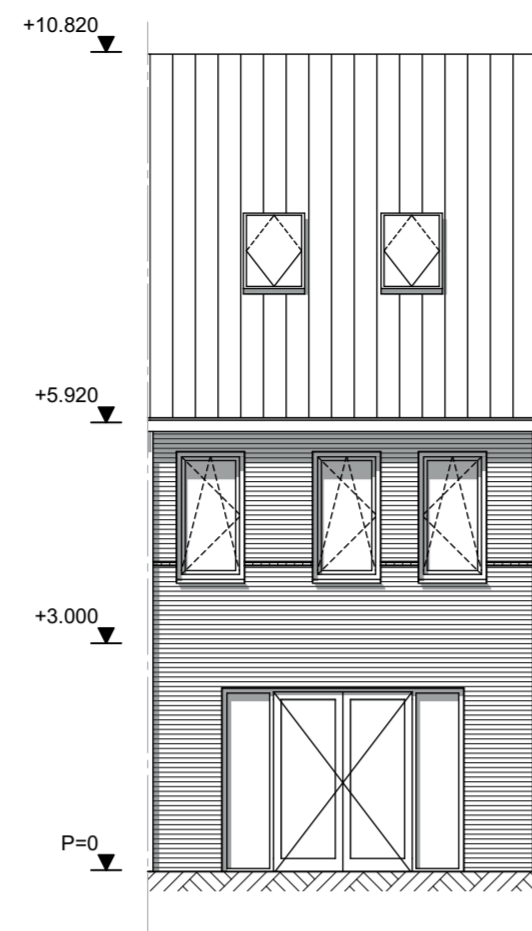
Achtergevel
