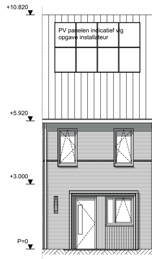
Voorgevel
