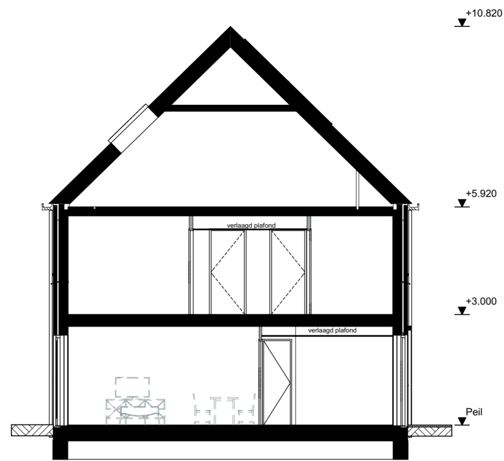
Doorsnede
