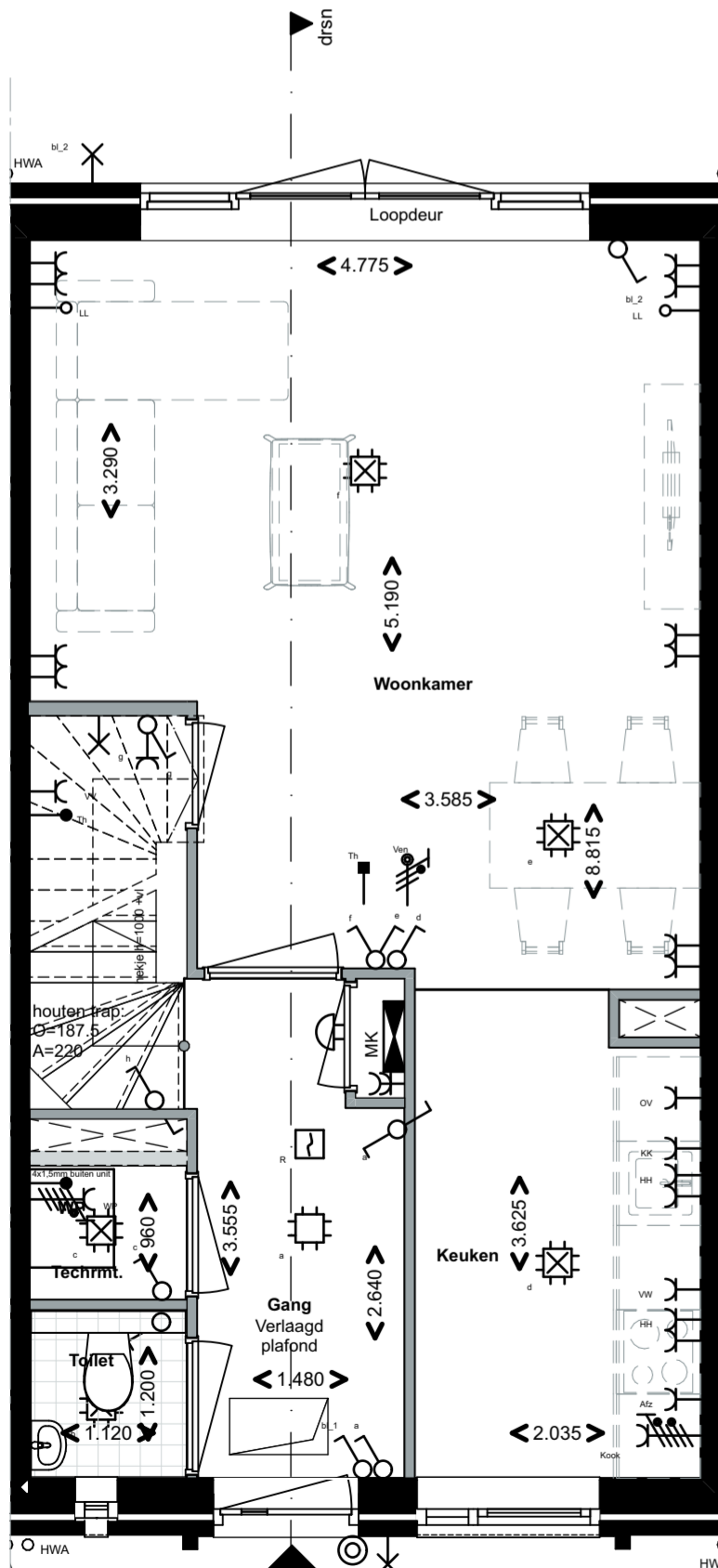
Begane grond
