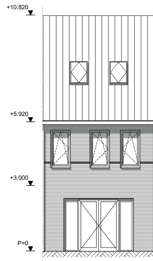
Achtergevel
