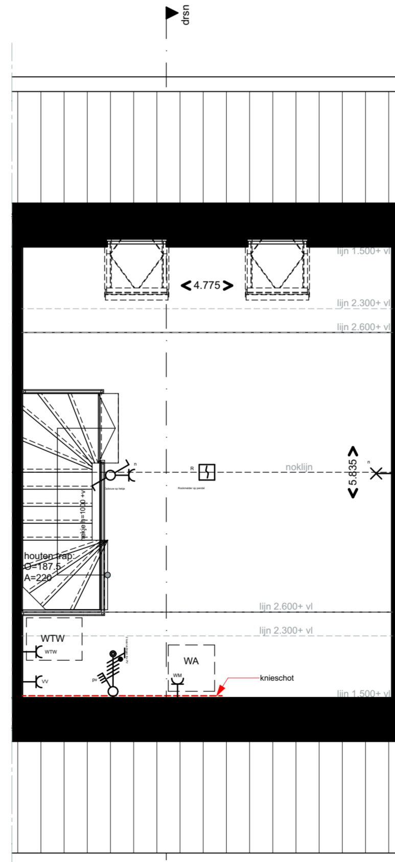
Tweede verdieping
