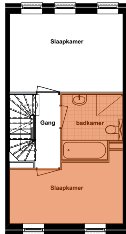
Eerste verdieping optionele indeling vergrote badkamer
